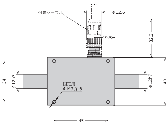
キー溝オプション：UTMII-5/10Nm(K)
