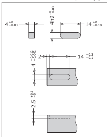
キー溝オプション：UTMII-5/10Nm(K)
