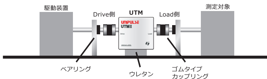
<推奨するカップリングの取り付け方>
