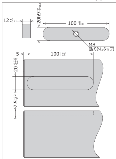
キー溝オプション : UTM II-2000Nm(K)
